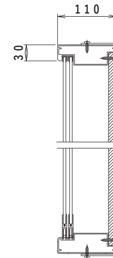
A-A断面図 (1:5)
