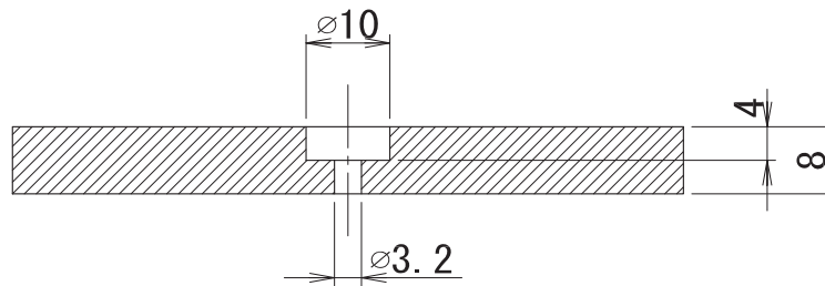
A-A断面詳細
