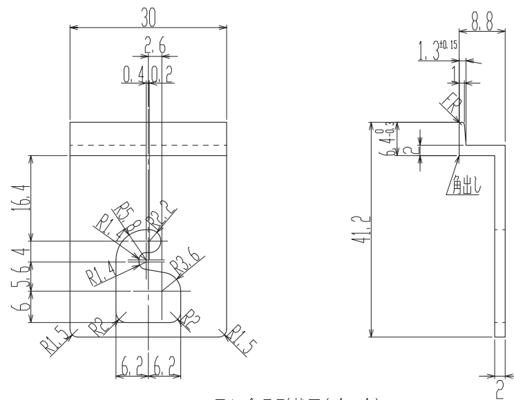
吊り金具形状図(1:1)
