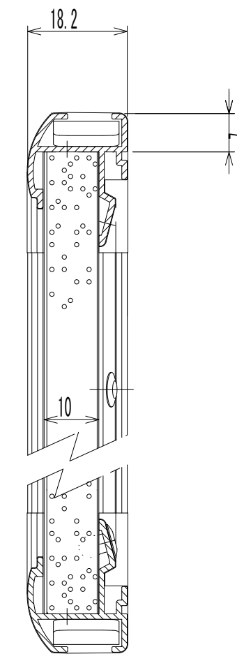
ボード断面図 (1/1)
