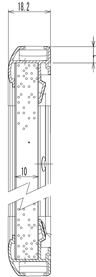
ボード断面図 (1/1)
