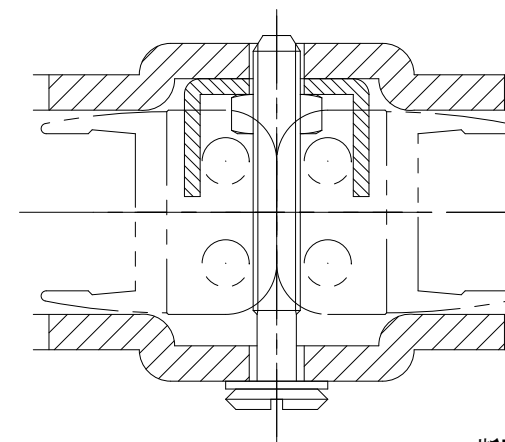
A-A断面詳細 (1/1)
