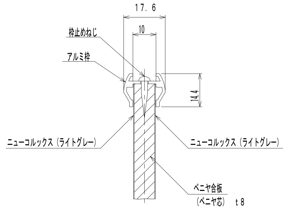
ボード断面図 (1/1)
