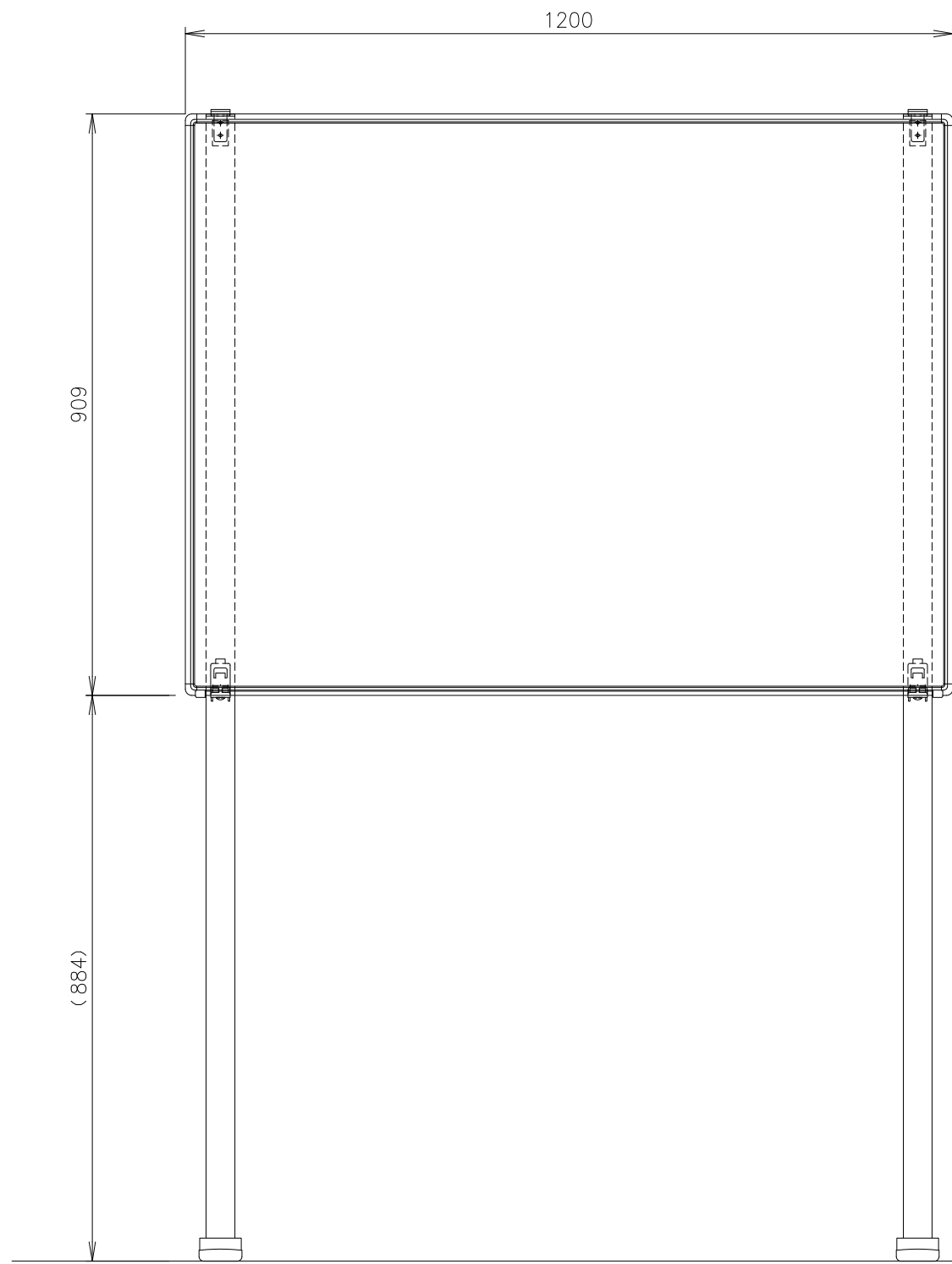
正面 1 : 10
