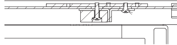
断面図 C-C スケール 1:2
