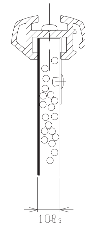
掲示板枠固定金具 取付部詳細 (1/1)
